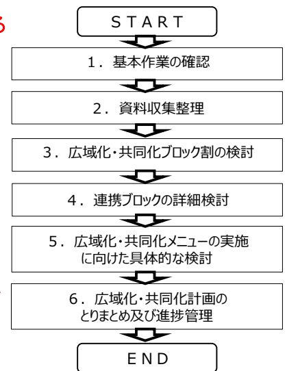
図2-1. 作業フロー
